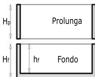
SEZIONE
